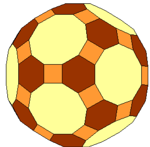
abgestumpftes Ikosidodekaeder
