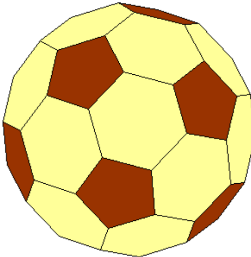
abgestumpftes Ikosaeder
