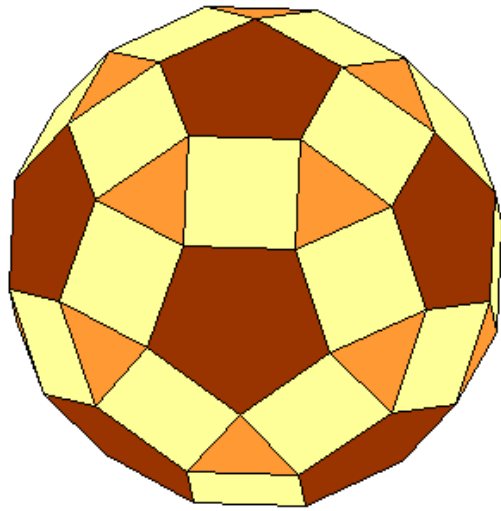
Rhombenikosidodekaeder
