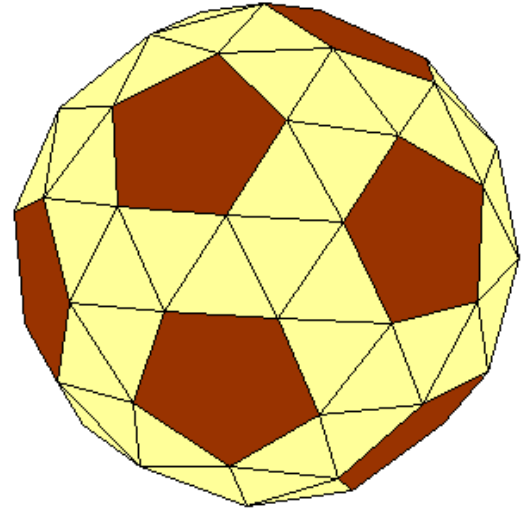
abgeschrägtes Dodekaeder
